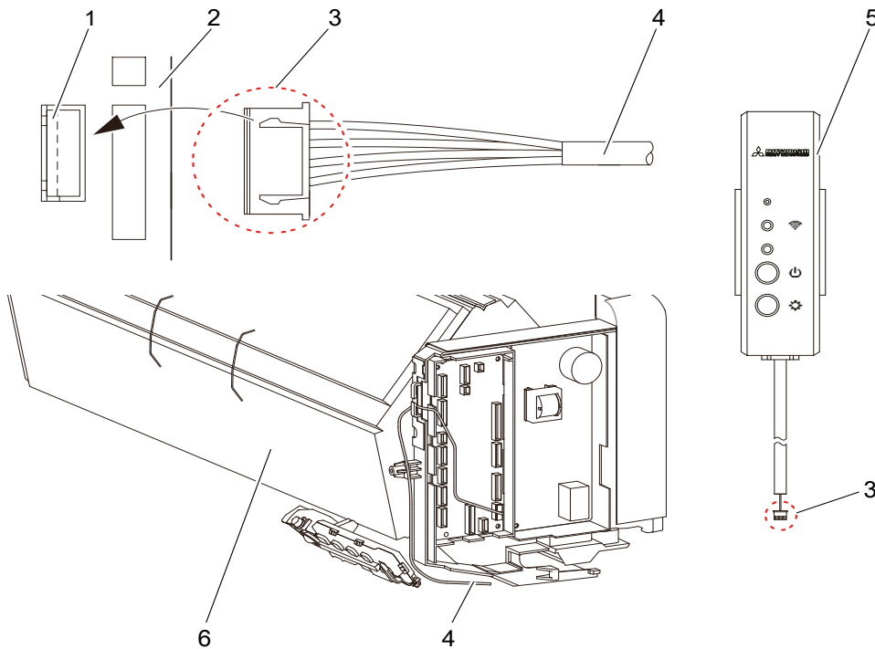
Abbildung 6: Anschluss des WLAN-Adapters an das Innengerät
